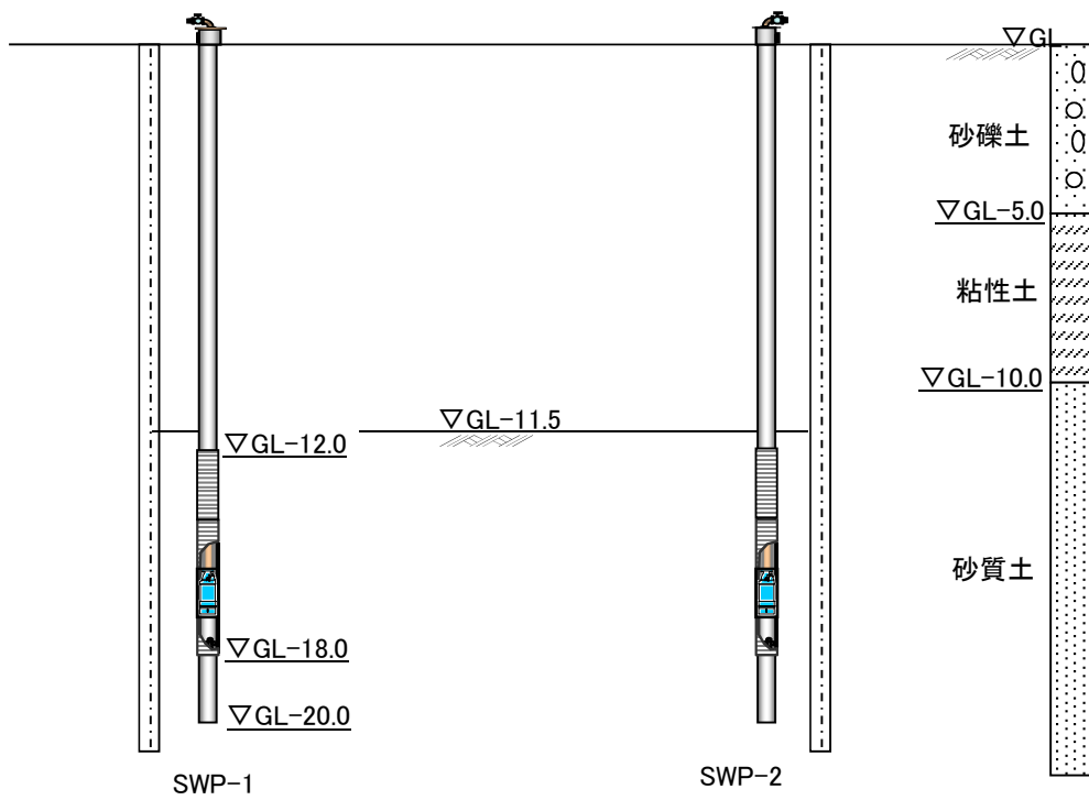
断面図
